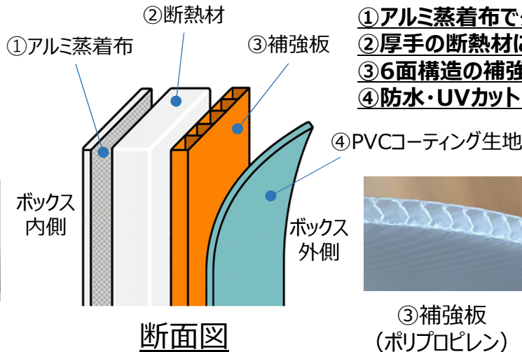
②断熱材 (発泡ポリエチレン)
